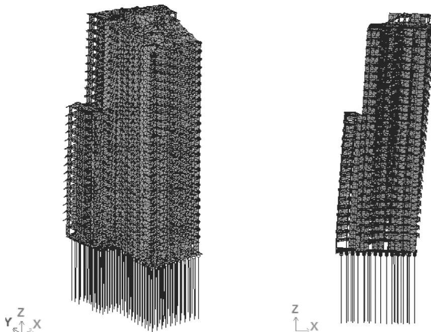
Рис. 5. Деформована схема будівлі при лінійному розрахунку (тип 1)
