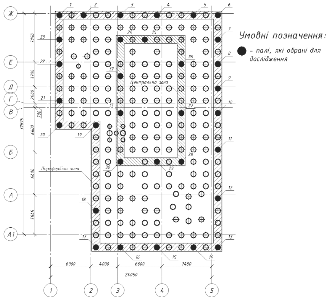
Рис. 4. Схема розміщення палей з зонами дослідження
