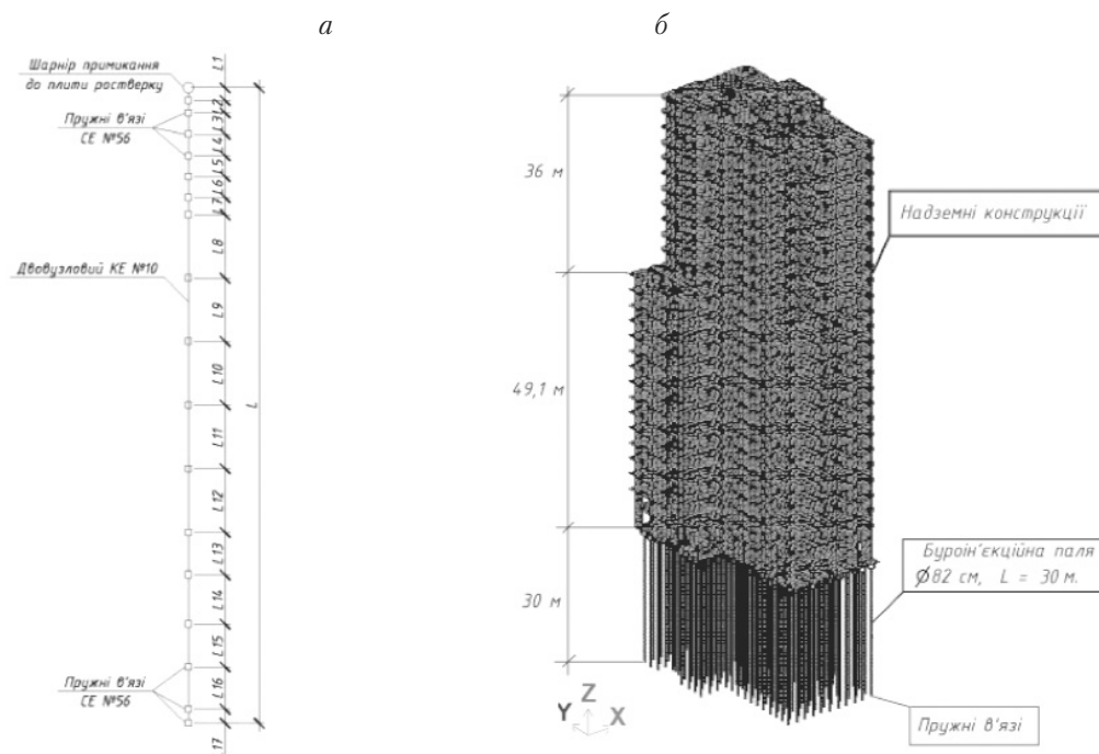
Рис. 2. Скінченно-елементна модель для лінійного розрахунку з використанням пружних в'язей (тип 1) а — модель палі; б — модель всієї будівлі
