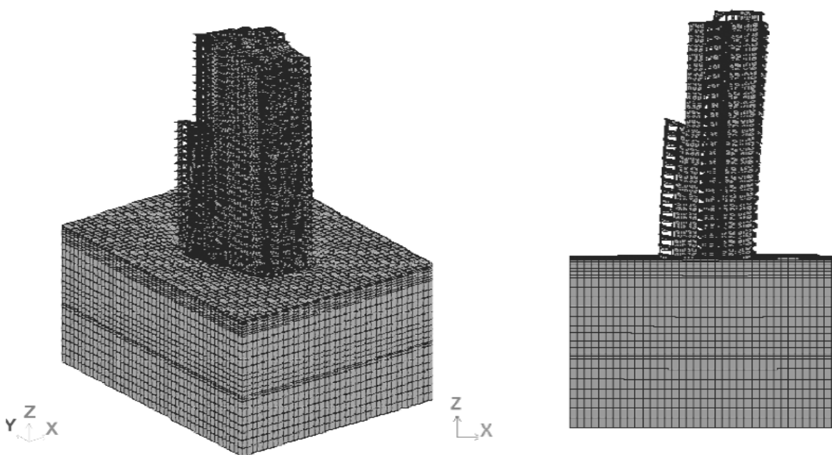
Рис. 7. Деформована схема будівлі при нелінійному розрахунку (тип 3)
