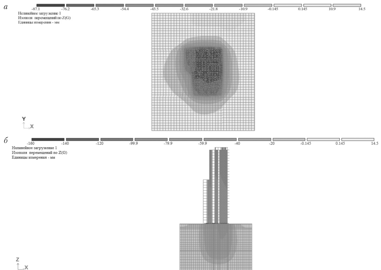
Рис. 9. Изополя перемещений грунта в направлении Z при нелинейном расчете (тип 3): а — в уровне подошвы плитного ростверка; б — поперечный разрез
